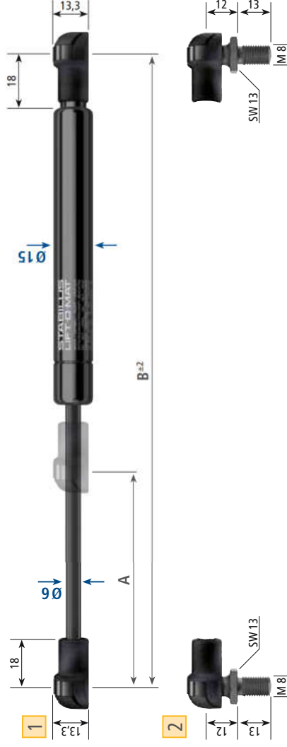
Suitable for ball studs according to DIN 71803 Ø 10 Passend für Kugelzapfen nach DIN 71803 Ø 10
