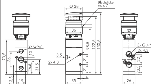
5/2-Wege Pilztaster
