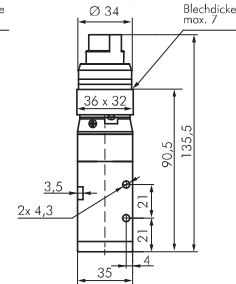
5/2-Wege Drehschalter
