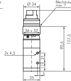
3/2-Wege Drehschalter
