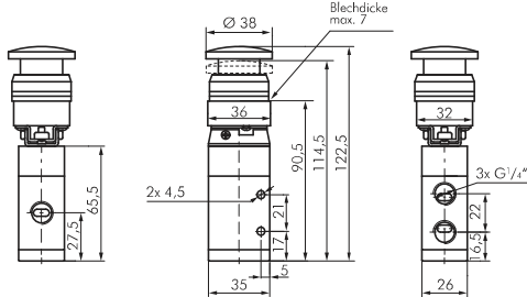
3/2-Wege Pilztaster
