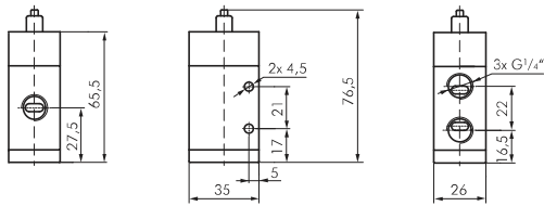
5/2-Wege Nockenventil
