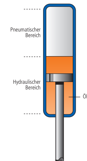
Hydraulische Dämpfung
