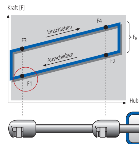
Federkennlinie und F1-Kraft
