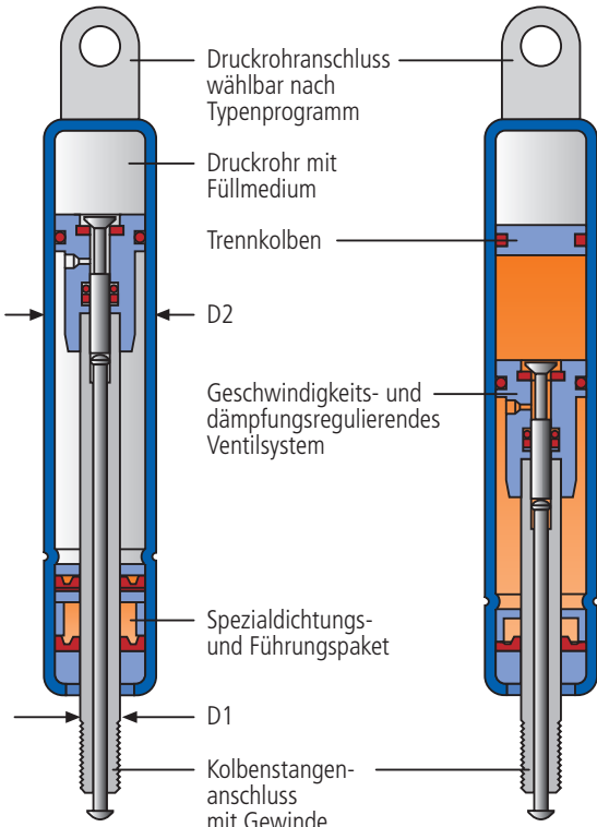
Links: Federnd blockierbare BLOC-O-LIFT® Gasfeder Rechts: Starr blockierbare BLOC-O-LIFT® Gasfeder mit Trennkolben für lageunabhängigen Einbau
