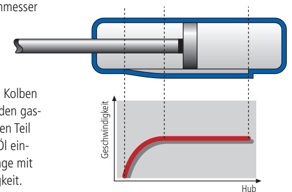
Dynamische Dämpfung
